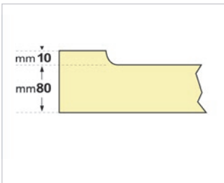
Detalle del panel de suelo. Perfil sanitario de 1 mm de radio.
