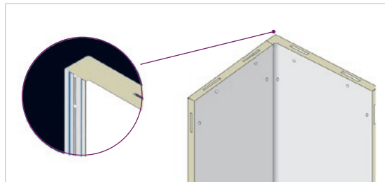
Sin necesidades de angula res. Los paneles disponen ya de un ángulo que facilita la instalación.
