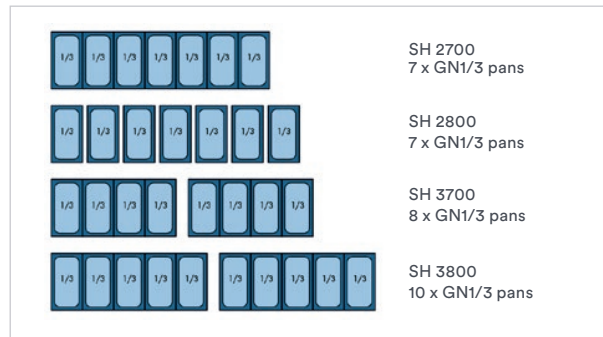
Distribución de cubetas modelos SH
