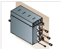
Instalación vertical Instale la unidad con la caja de control mirando hacia arriba.
