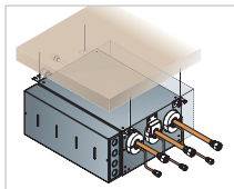
Instalación en techo Desde el techo se instala en posición horizontal.
